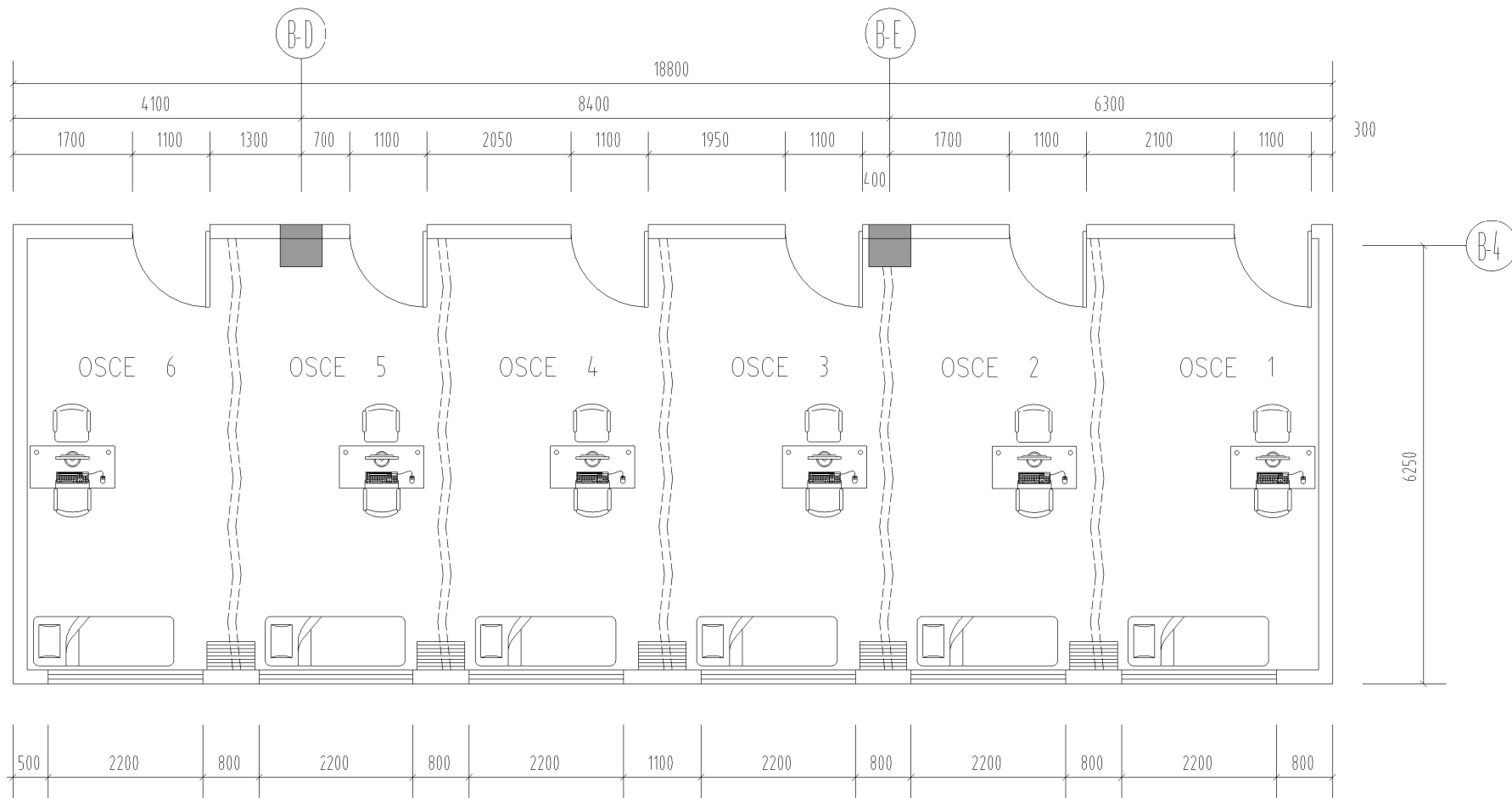
0' DETAIL OSCE室平面图 -- SCALE 1:45
